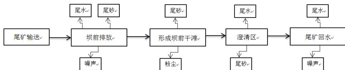
图 3.2-4 运行期产污环节示意图
