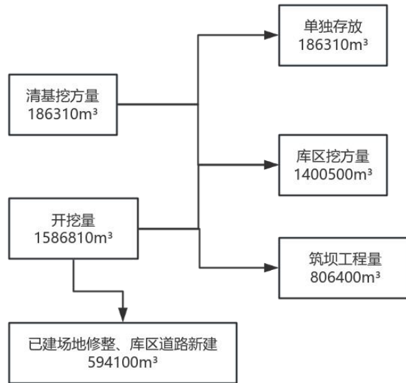
图 3.2-2 土石方平衡图
