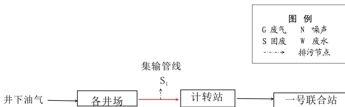
图 3.3-4 油气集输工艺流程图
