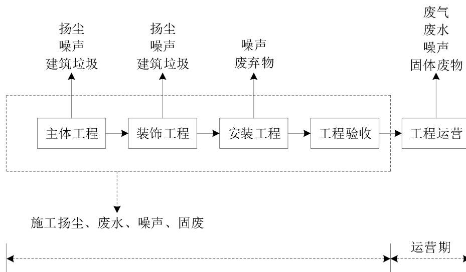
图 2.3-1 项目施工期工艺流程及产物节点图
