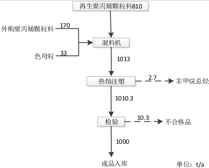
图2.4-5 周转筐生产物料平衡图
