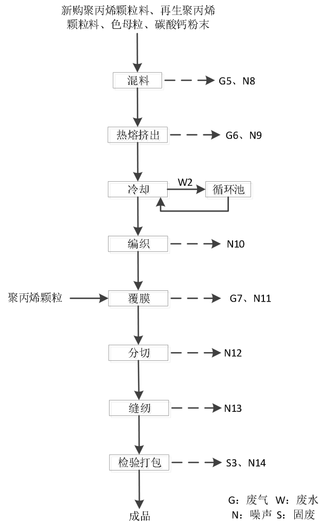
图2.3-4 铝用打包袋生产工序工艺流程及产污环节图
