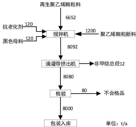
图2.4-1 滴灌带生产物料平衡图
