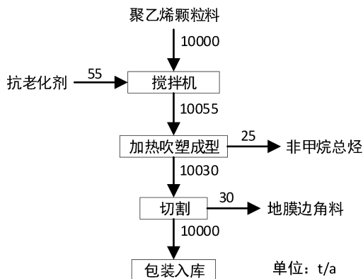
图2.4-2 地膜生产物料平衡图
