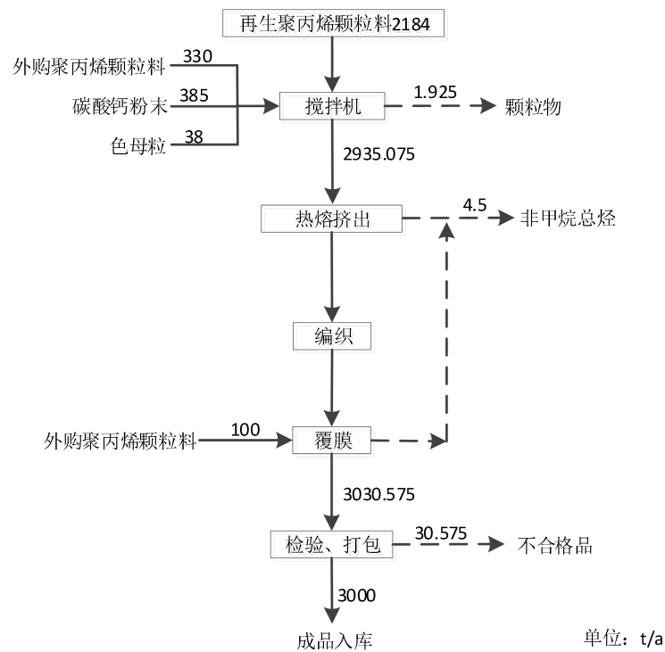
图2.4-3 铝用打包带生产物料平衡图
