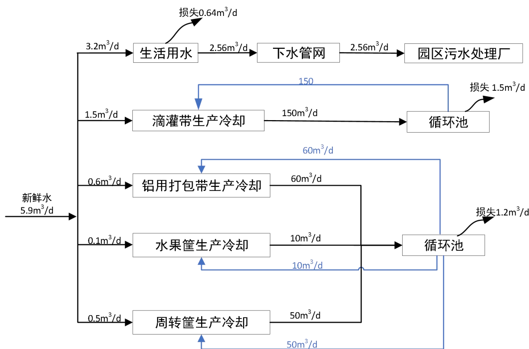
图2.5-6 项目水平衡图
