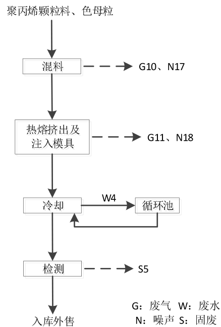
图2.3-6 水果筐生产工艺流程及产污环节图
