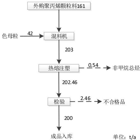
图2.4-4 水果筐生产物料平衡图
