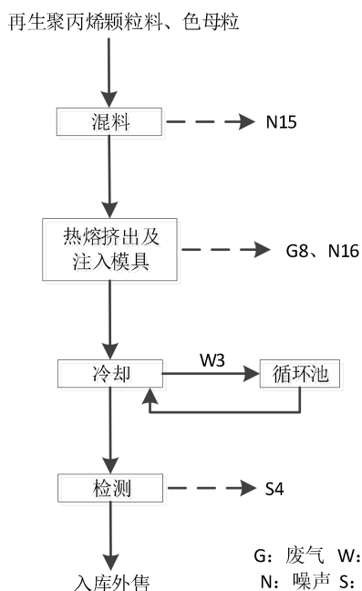
图2.3-5 周转筐生产工艺流程及产污环节图
