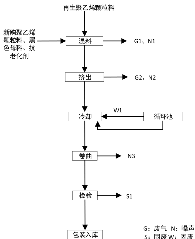
图2.3-2 滴灌带及水带生产线工艺流程及产污环节图
